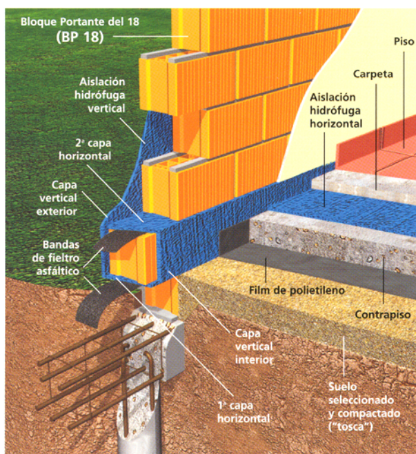
El dado hidrófugo
