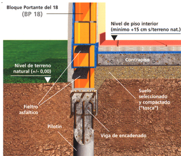
Fundación con pilotes y vigas de encadenado
