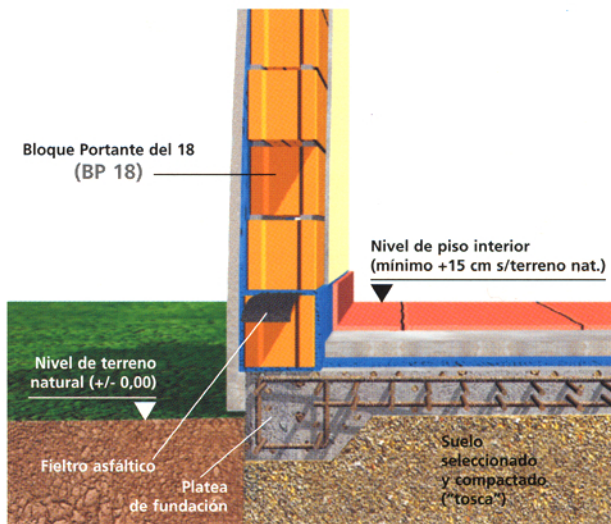
Fundación con platea
