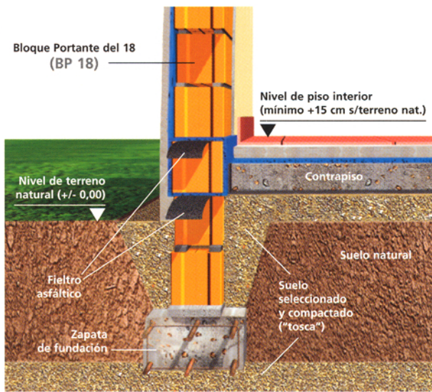
Fundación con zapata corrida
